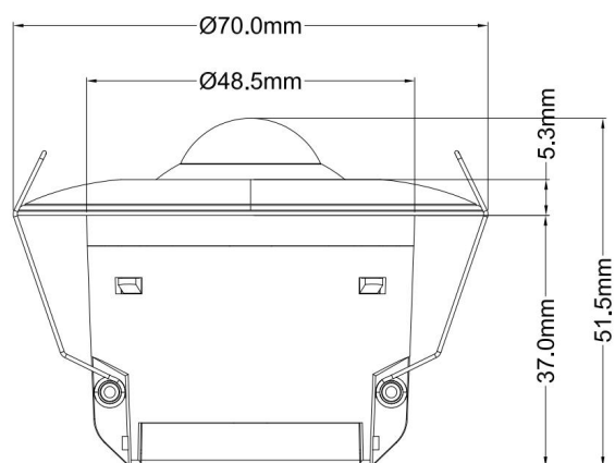
CSBP-04/00.1.0x and CSBP-04/00.2.0x
