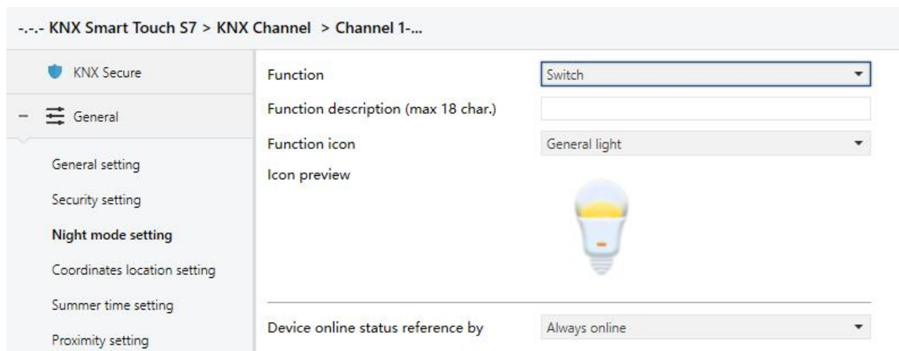
Fig.5.11.2(1) "Switch"parameter window
