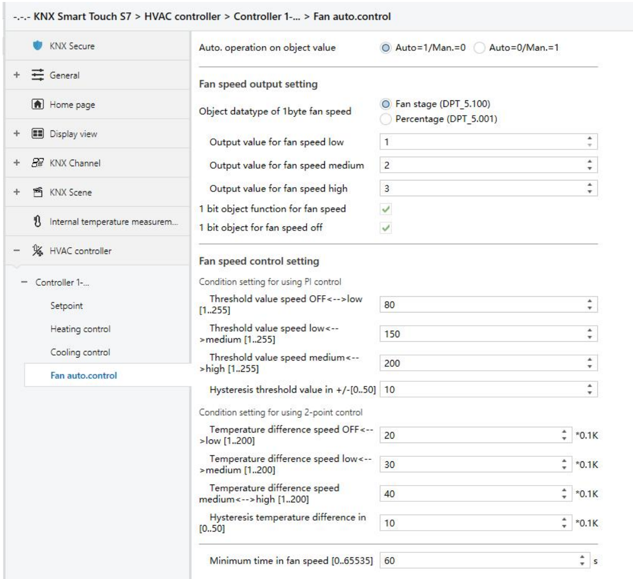
Fig.5.3.1.3"Fan" parameter window
